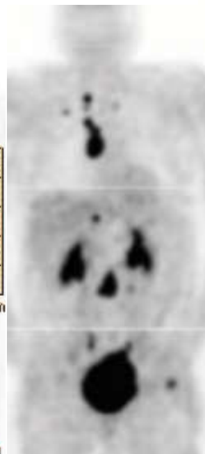
18F DOPA
