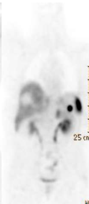
68Ga DOTATOC
