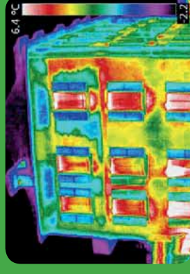
Thermographie infrarouge d'un bâtiment
